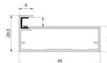
Профиль 45 мм сечение
